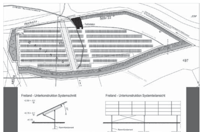
Bild: Modulbelegung sowie Systemschnitt mit Höhenangaben
