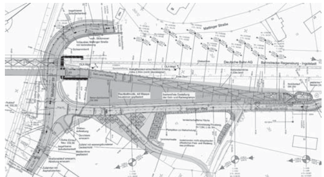
Auszug aus Unterlage 5.2_1 (Lageplan) NORD (Seite Regensburg) ohne Maßstab
