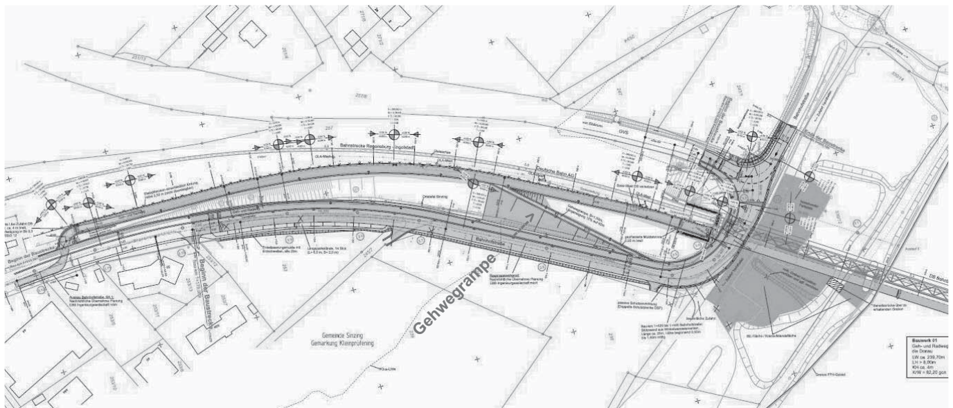
Auszug aus Unterlage 5.1_1 (Lageplan) SÜD (Seite Sinzing)
