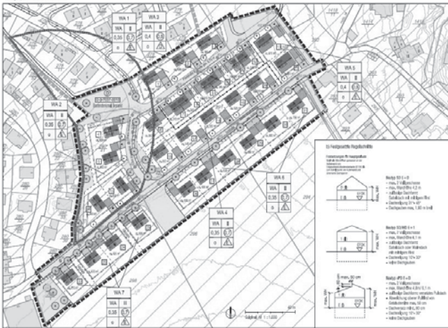
Vorläufiger Baueckelplan mit integriertem Grünordnungsplan Lageplan M 1:1000
