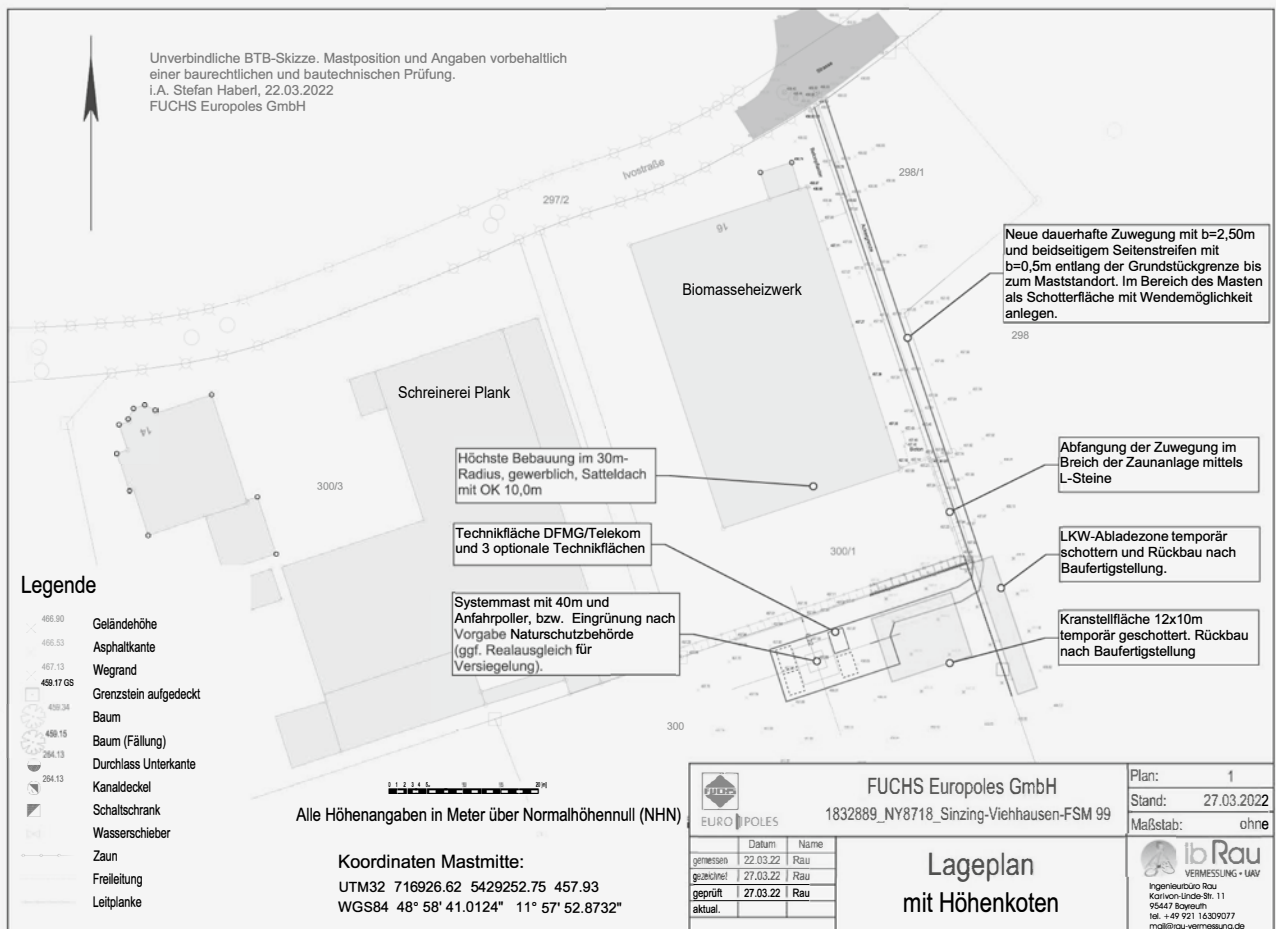
Der Mobilfunkmast soll direkt hinter dem Biomasseheizwerk gebaut werden.
